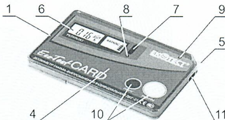
Рисунок 1 – Зовнішній вигляд дозиметра ДКГ-21 спереду
