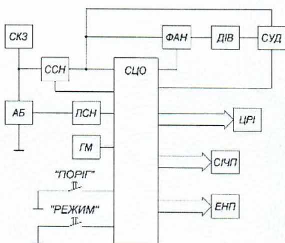
Рисунок 7 – Структурна схема дозиметра ДКГ-21.
