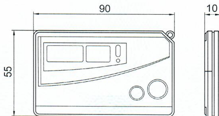
Рисунок 3 – Габаритні розміри дозиметра ДКГ-21
