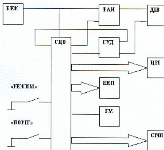
Рисунок 8 – Структурна схема дозиметра ДКГ-21М.
