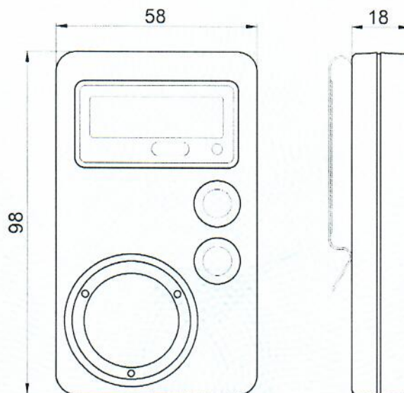
Рисунок 5 – Габаритні розміри дозиметра ДКГ-21М
