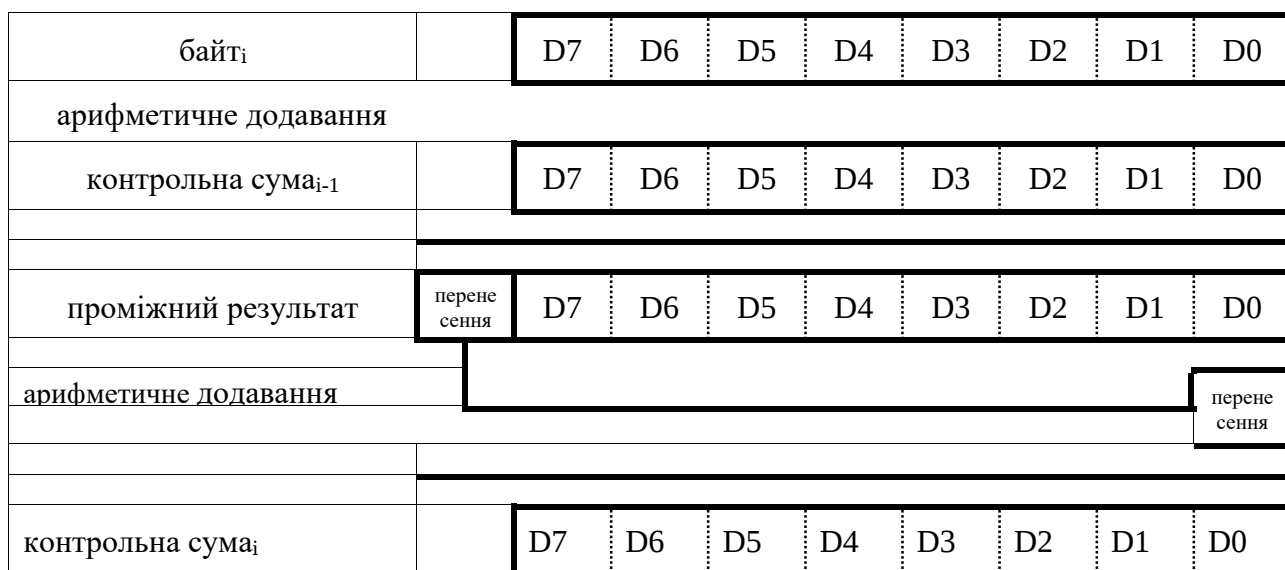
Рисунок Б.1 - Алгоритм підрахунку контрольної суми
