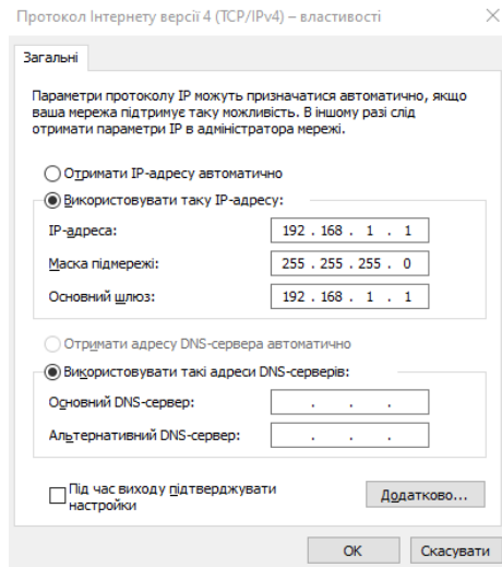
Рисунок Ж.1 – Властивості протоколу інтернету версії 4 (TCP/IPv4)
